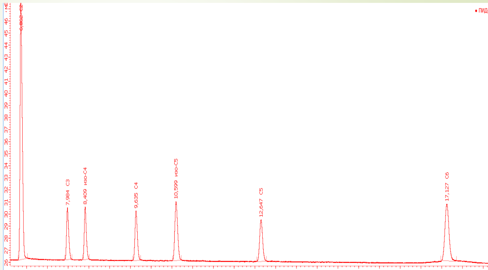
Хроматограмма модельной смеси КЦЖК
